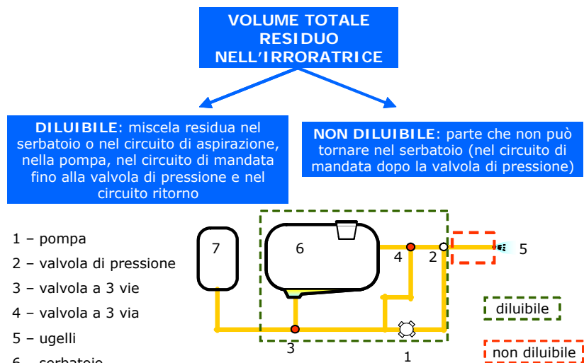
Fig. 41 – Residuo a fine trattamento: differenza tra frazione diluibile e non diluibile.
