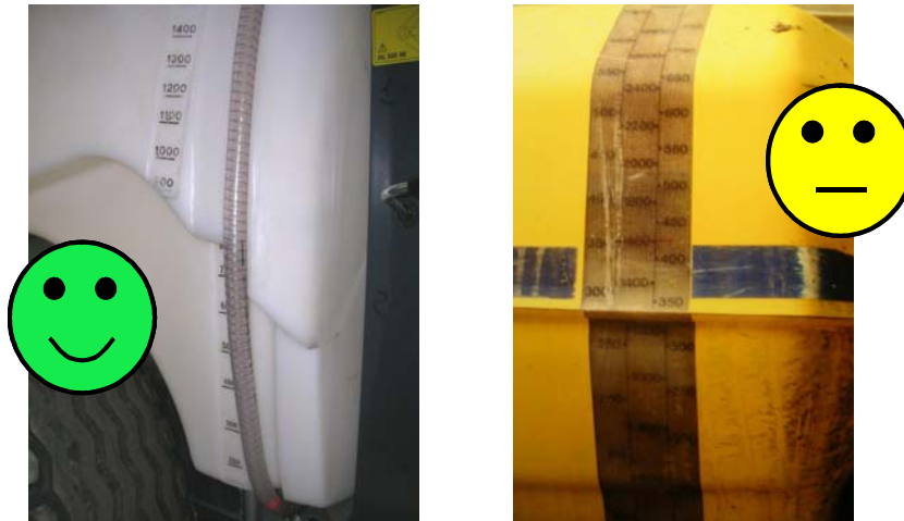
Fig. 56 - Una indicazione precisa e leggibile del liquido presente nel serbatoio è indispensabile per poter inserire nel serbatoio stesso il volume di acqua desiderato.
