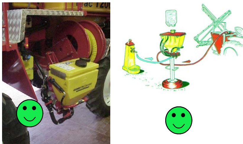
Fig. 67 – I premiscelatori possono essere montati direttamente sull'irroratrice (sinistra) oppure indipendenti (destra) ed alimentati direttamente dalla rete idrica dell'acquedotto.
