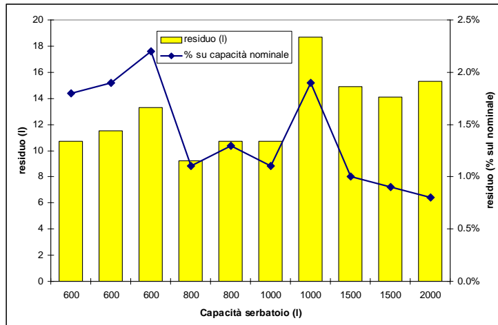
Fig. 40 – Alcuni esempi di quantità di miscela residua nel serbatoio (residuo diluibile) di differenti modelli di irroratrici per colture arboree (prove DEIAFA).
