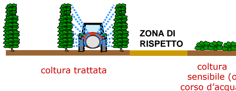
Fig. 80 - Le zone di rispetto (buffer zones) servono a preservare colture sensibili o corsi d'acqua dal rischio di essere contaminati dalla miscela fitoiatrica che si sta distribuendo.
