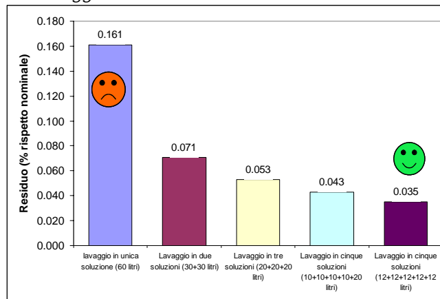
Fig. 91 - Ottimizzazione del lavaggio interno mediante successivi risciacqui ottenuti frazionando l'acqua pulita del lavapianto (prove DEIAFA)
