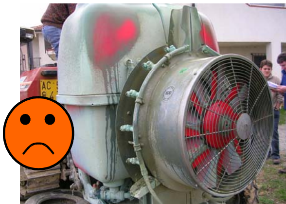
Fig. 38 - Esempio di macchina irroratrice in cui il getto erogato colpisce il serbatoio determinando il gocciolamento a terra della miscela fitoiatrica e causando, quindi, inquinamento puntiforme.
