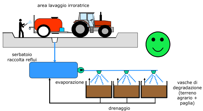
Fig. 95 - Raccolta delle acque reflue del lavaggio e loro biodegradazione (biobac ®). Il contenuto delle vasche di degradazione viene monitorato e periodicamente arieggiato e rivoltato e deve essere sostituito ogni circa 5 anni. Tale terreno esausto può poi essere distribuito in campo
